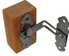
Fransız Kilidi (90 Derece)
